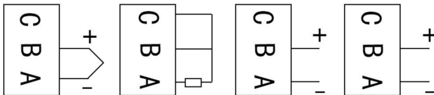
热电偶 信号接入
